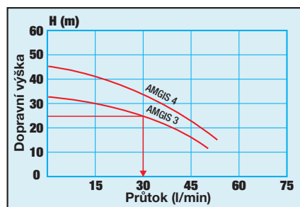
Diagram výkonu zařízení AMGIS
