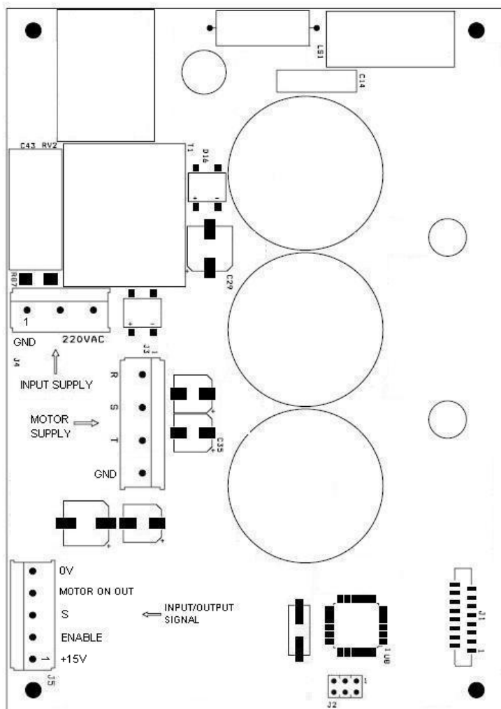
Obrázek 14: Elektronický panel typu IMMP-IMTP
