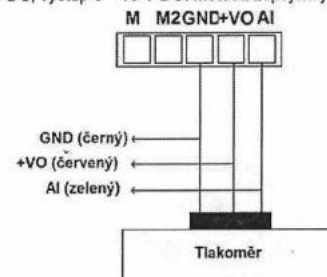
Schéma zapojení tlakoměru
