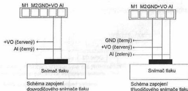
Schéma zapojení tlakoměru
